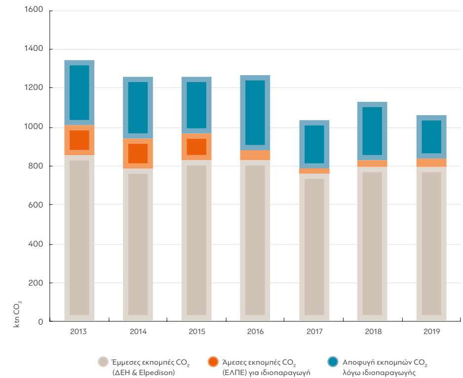
Συμβολή της ιδιοπαραγόμενης ηλεκτρικής ενέργειας στα διυλιστήρια του Ομίλου και εκπομπές CO 2 που αποφεύχθηκαν λόγω της ιδιοπαραγόμενης ηλεκτρικής ενέργειας σε συνάρτηση με αυτές της συνολικής κατανάλωσης
