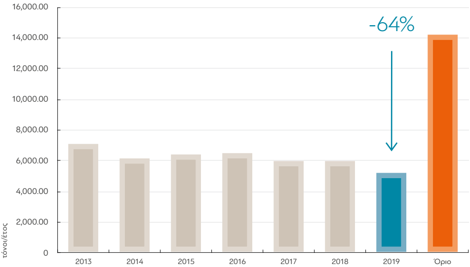
Σύγκριση εκπομπών Διοξειδίου του Θείου (SO 2 ) 2013-2019 με το ισχύον όριο
