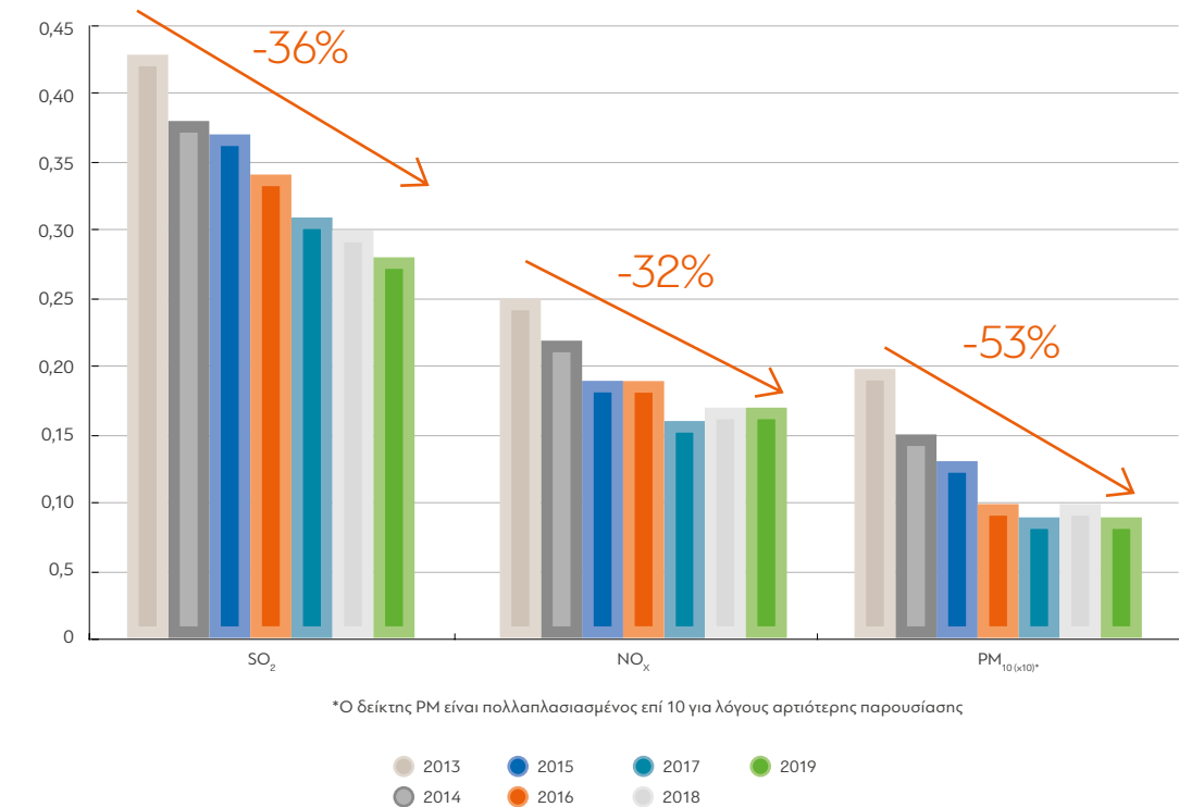
Δείκτες για τις Εκπομπές Διοξειδίου του Θείου (SO 2 ), Οξειδίων του Αζώτου (NO x ) και Σωματιδίων (PM 10 ) (kg εκπομπών ανά τη τροφοδοσίας από 2013 έως 2019)
